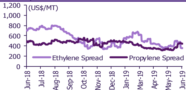
Olefins spreads
